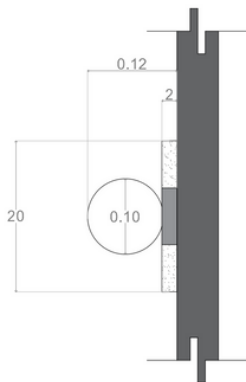
Alzado lateral
