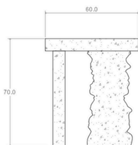
Alzado 01
