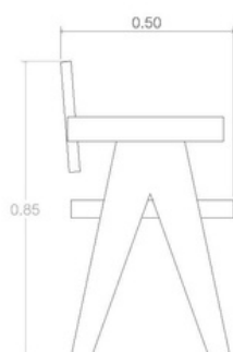
Alzado lateral
