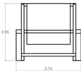
Alzado frontal
