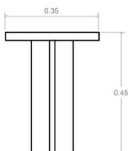
Alzado 01
