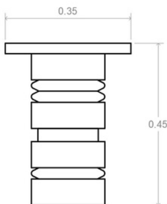
Alzado
